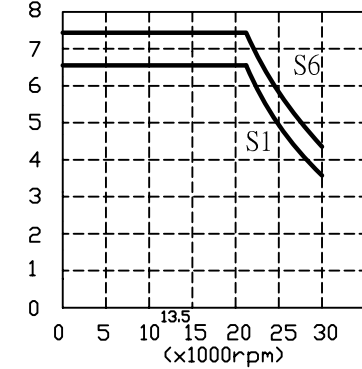
(Nm) Torque-diagram
