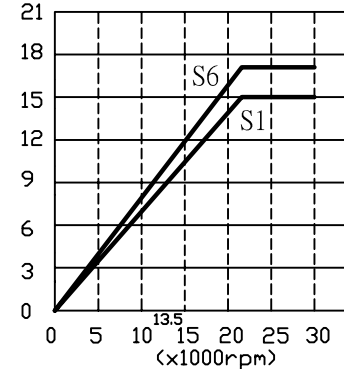
(kw) Power-diagram
