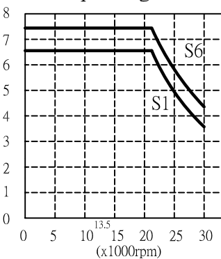
(Nm) Torque-diagram
