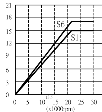
(kW) Power-diagram
