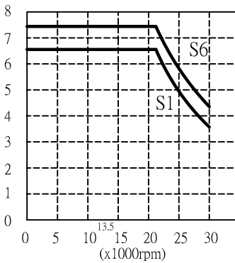
(Nm) Torque-diagram
